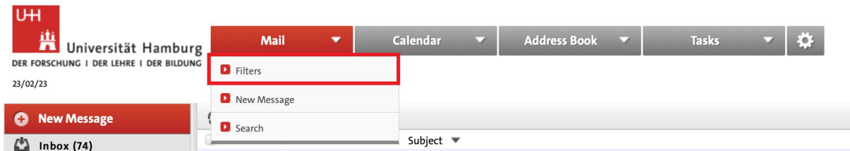
Fig. 5 Surfmail
