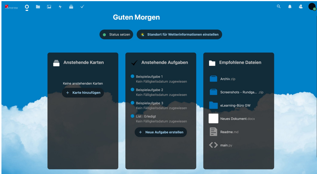
Fig. 14 UHH-Cloud
