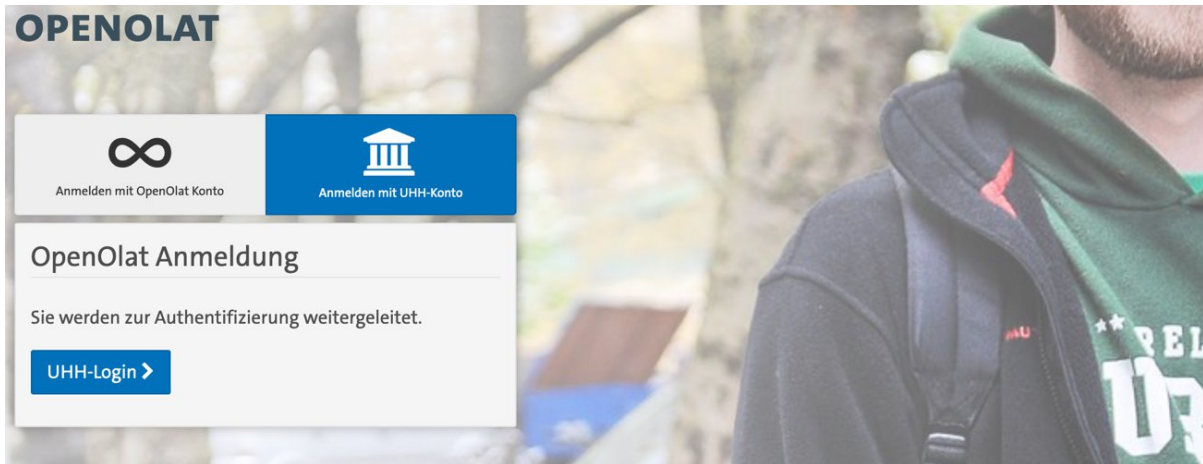
Fig. 9 OpenOlat Login
