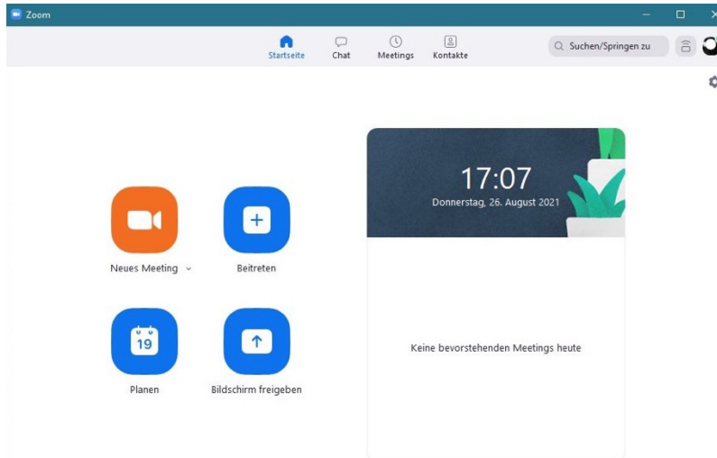
Fig. 11 Zoom-Client
